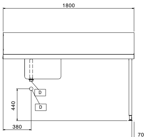
Zij aanzicht
